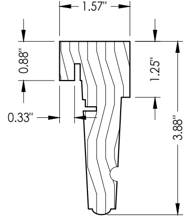
45 ASTRAGAL
